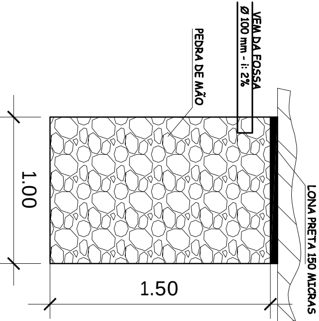
SUMIDOURO - EM ELEVAÇÃO
